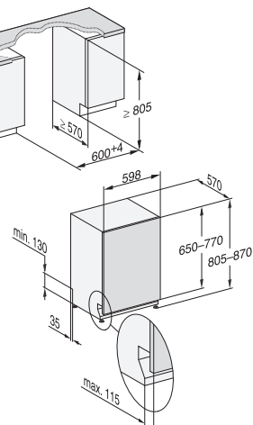
G 1xxxx-60 / PFD 10x-60, entièrement intégrable
