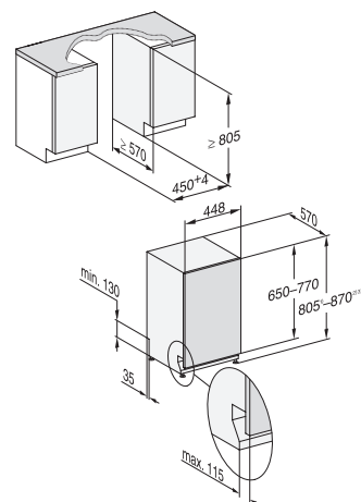
G 15xxx-45, entièrement intégrable
