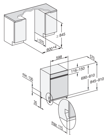
PFD 104-60, entièrement intégrable
