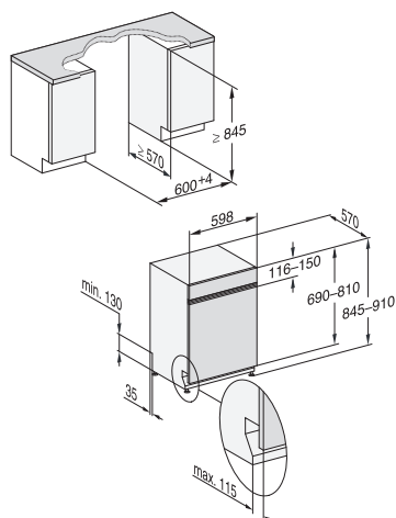
G 1xxxx-60 / PFD 10x-60, intégrable
