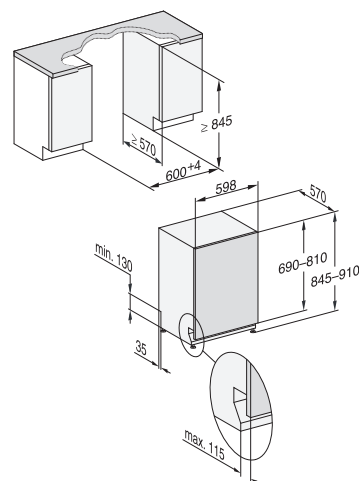
G 2xxxx-60 XXL / PFD 10x-60 XXL, entièrement intégrable
