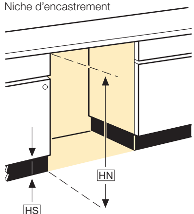
Niche d'encastrement
