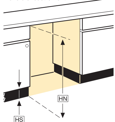
Niche d'encastrement
