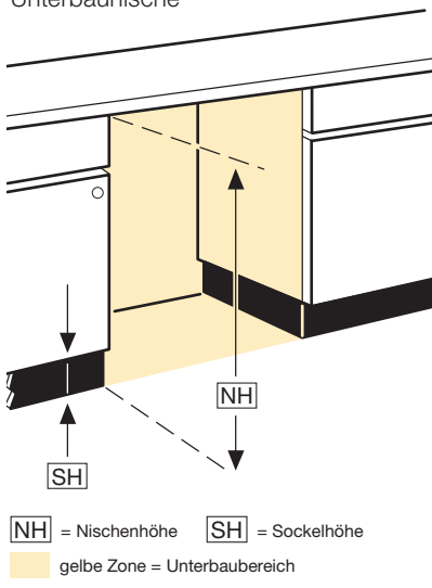
Unterbaunische
