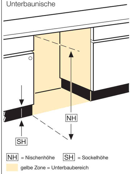
Unterbaunische
