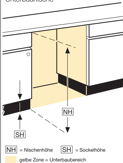
Unterbaunische
