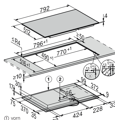
Induktionskochfeld KM 7515 FX, flächenbündig
