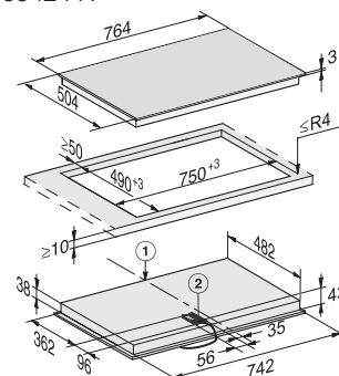
Elektrokochfeld KM 6542 FR
