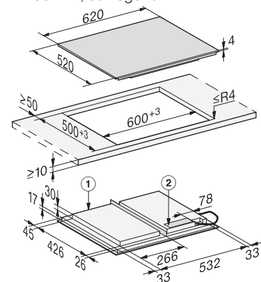
Induktionskochfeld KM 7667 FL, aufliegend
