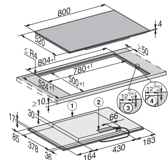
Induktionskochfeld KM 7474 FL, flächenbündig
