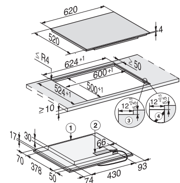
Induktionskochfeld KM 7464 FL, flächenbündig
