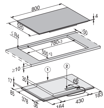
Induktionskochfeld KM 7474 FL, aufliegend
