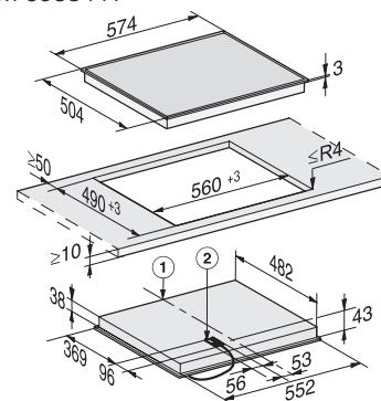
Elektrokochfeld KM 6538 FR
