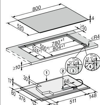
Induktionskochfeld KM 7679 FL, flächenbündig
