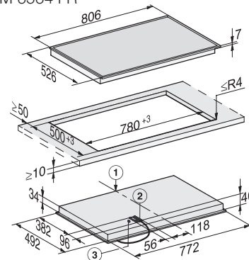
Elektrokochfeld KM 6564 FR
