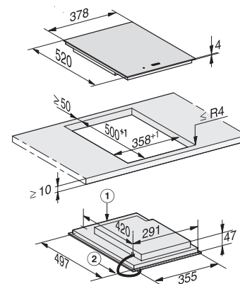
Induktionskochfeld CS 7612 FL, aufliegend
