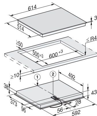
Elektrokochfeld KM 6540 FR
