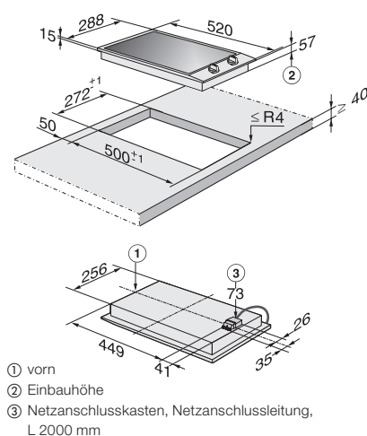
Induktionskochfeld CS 1212-1 I
