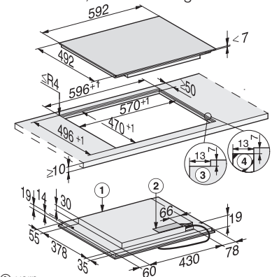
Induktionskochfeld KM 7404 FX, flächenbündig
