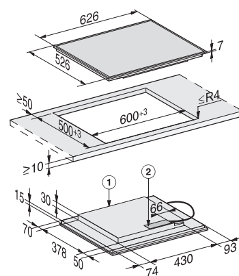
Induktionskochfeld KM 7564 FR
