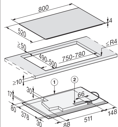
Induktionskochfeld KM 7679 FL, aufliegend
