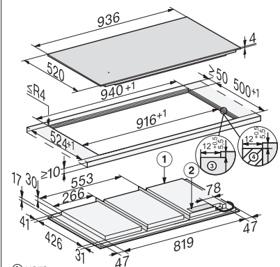
Induktionskochfeld KM 7897 FL, flächenbündig
