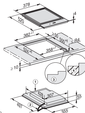
Teppan Yaki Induktion CS 7632 FL, flächenbündig
