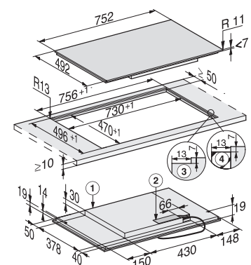
Induktionskochfeld KM 7414 FX, flächenbündig
