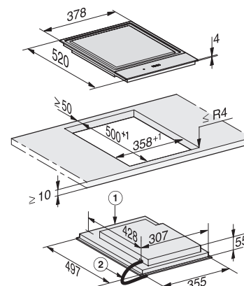
Teppan Yaki Induktion CS 7632 FL, aufliegend
