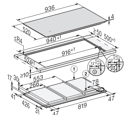
Induktionskochfeld KM 7697 FL, flächenbündig
