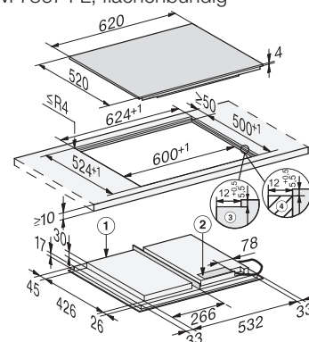
Induktionskochfeld KM 7867 FL, flächenbündig
