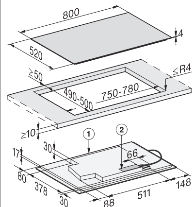
Induktionskochfeld KM 7879 FL, aufliegend
