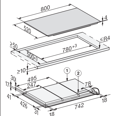
Induktionskochfeld KM 7678 FL, aufliegend
