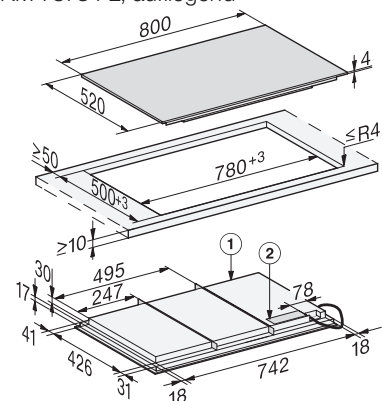
Induktionskochfeld KM 7878 FL, aufliegend
