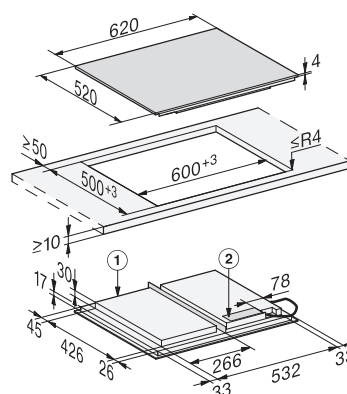
Induktionskochfeld KM 7867 FL, aufliegend
