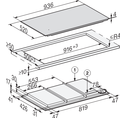
Induktionskochfeld KM 7697 FL, aufliegend
