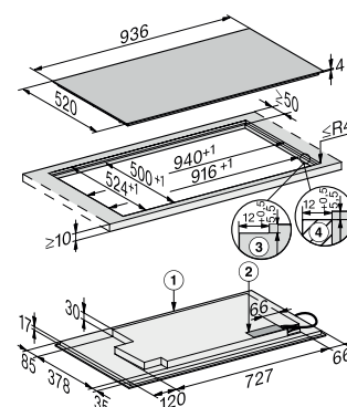
Induktionskochfeld KM 7899 FL, flächenbündig
