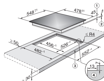
Kombinations-Elektrokochfeld KM 6017, flächenbündig
