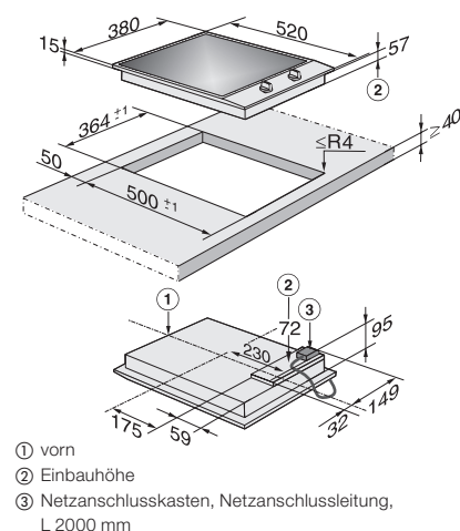
Elektrokochfeld CS 1122 E
