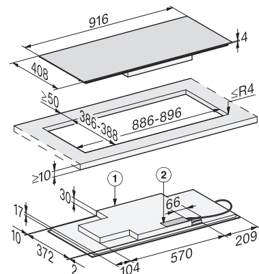
Induktionskochfeld KM 7689 FL, aufliegend
