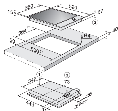
Induktionskochfeld CS 1221-1 I
