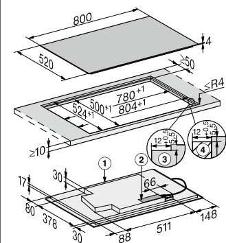
Induktionskochfeld KM 7879 FL, flächenbündig
