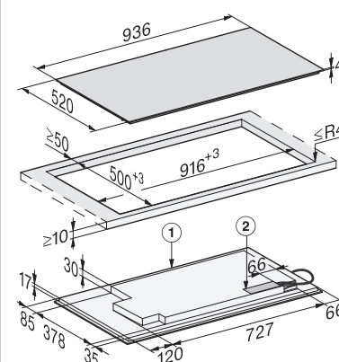
Induktionskochfeld KM 7899 FL, aufliegend
