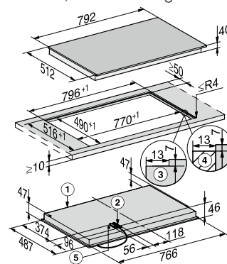
Elektrokochfeld KM 6564 FL, flächenbündig
