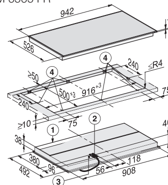
Elektrokochfeld KM 6565 FR
