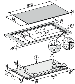
Induktionskochfeld KM 7629 FX, flächenbündig
