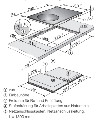
Induktionskochfeld KM 6359, flächenbündig
