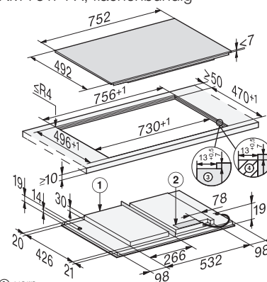
Induktionskochfeld KM 7617 FX, flächenbündig
