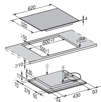
Induktionskochfeld KM 7564 FL, aufliegend
