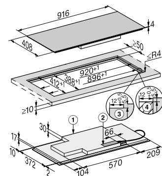
Induktionskochfeld KM 7689 FL, flächenbündig
