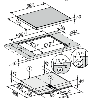
Elektrokochfeld KM 6539 FL, flächenbündig
