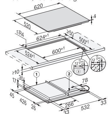
Induktionskochfeld KM 7667 FL, flächenbündig
