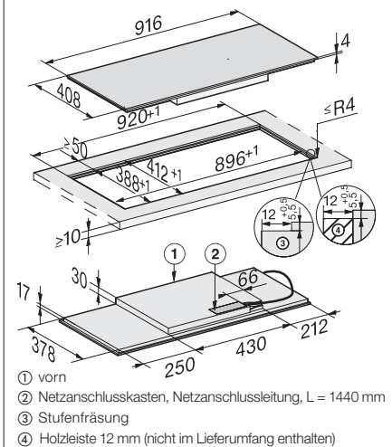
Induktionskochfeld KM 7684 FL, flächenbündig
