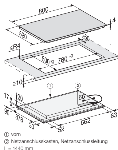
Induktionskochfeld KM 7575 FL, aufliegend
