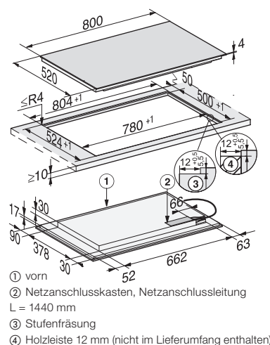
Induktionskochfeld KM 7575 FL, flächenbündig
