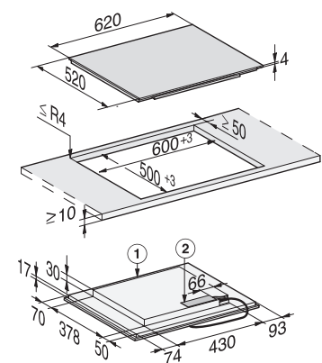
Induktionskochfeld KM 7464 FL, aufliegend
