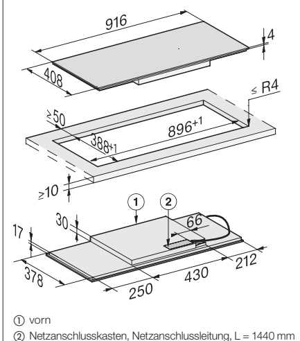
Induktionskochfeld KM 7684 FL, aufliegend
