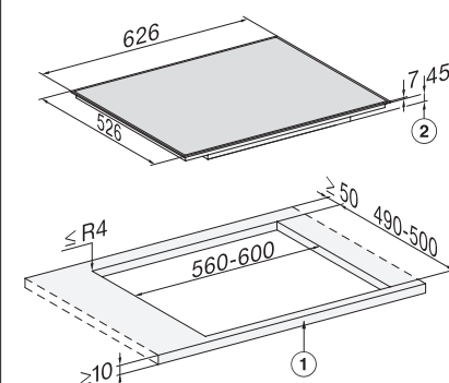
Kombinations-Induktionskochfeld KM 7005 FR
