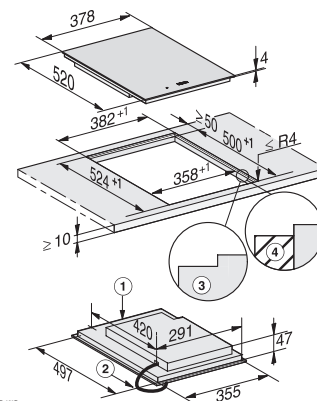
Induktionskochfeld CS 7612 FL, flächenbündig
