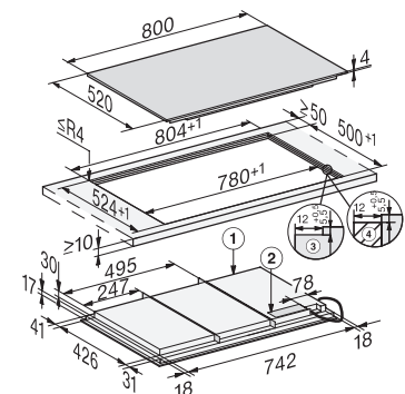
Induktionskochfeld KM 7878 FL, flächenbündig
