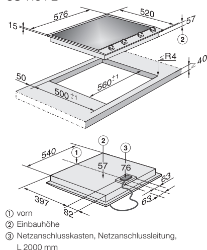
Elektrokochfeld CS 1134 E
