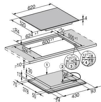
Induktionskochfeld KM 7564 FL, flächenbündig
