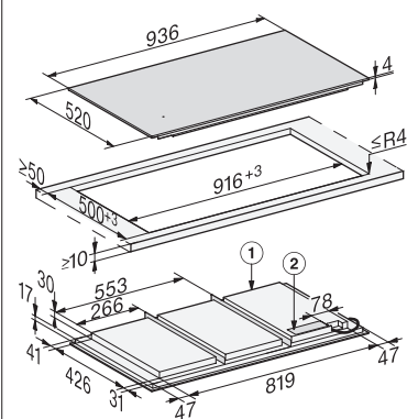
Induktionskochfeld KM 7897 FL, aufliegend
