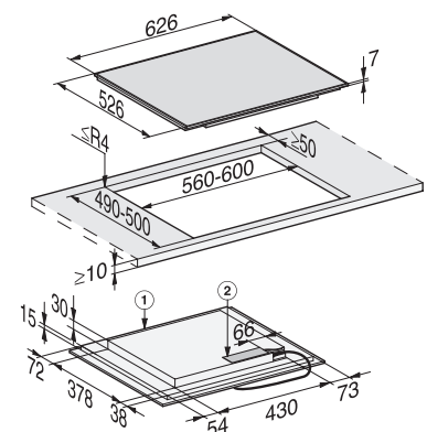
Induktionskochfeld KM 7464 FR
