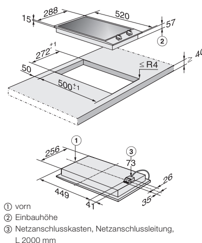
Elektrokochfeld CS 1112 E
