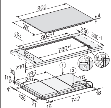
Induktionskochfeld KM 7678 FL, flächenbündig
