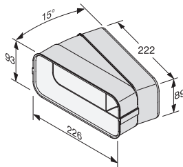
Courbe horizontale 15° DFK-BH 15
