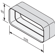
Pièce de raccordement au canal plat DFK-V ③
