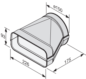
Adaptateur rectangulaire-rond DFK-A
