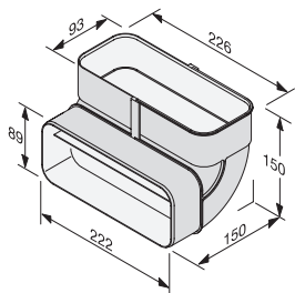
Courbe verticale 90° 150 mm DFK-BVK 90
