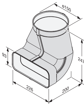
Adaptateur rectangulaire-rond 90° DFK-A 90
