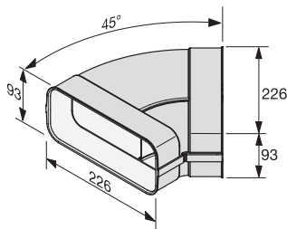
Courbe horizontale 45° DFK-BH 45
