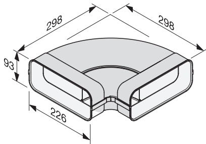
Courbe horizontale 90° DFK-BH 90 ④
